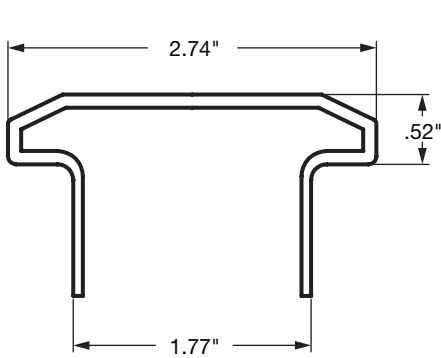
Rail Stiffener 018-7 $32.88/24'
