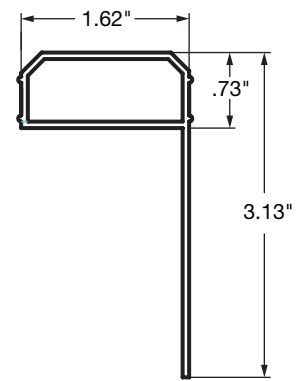
Rail Stiffener 018-3 $26.88/24'
