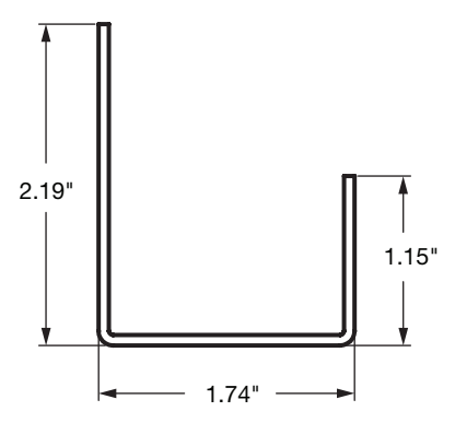
Post Stiffener 018-9 $20.88/24'
