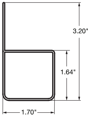
Rail Stiffener 018-4 $32.88/24'
